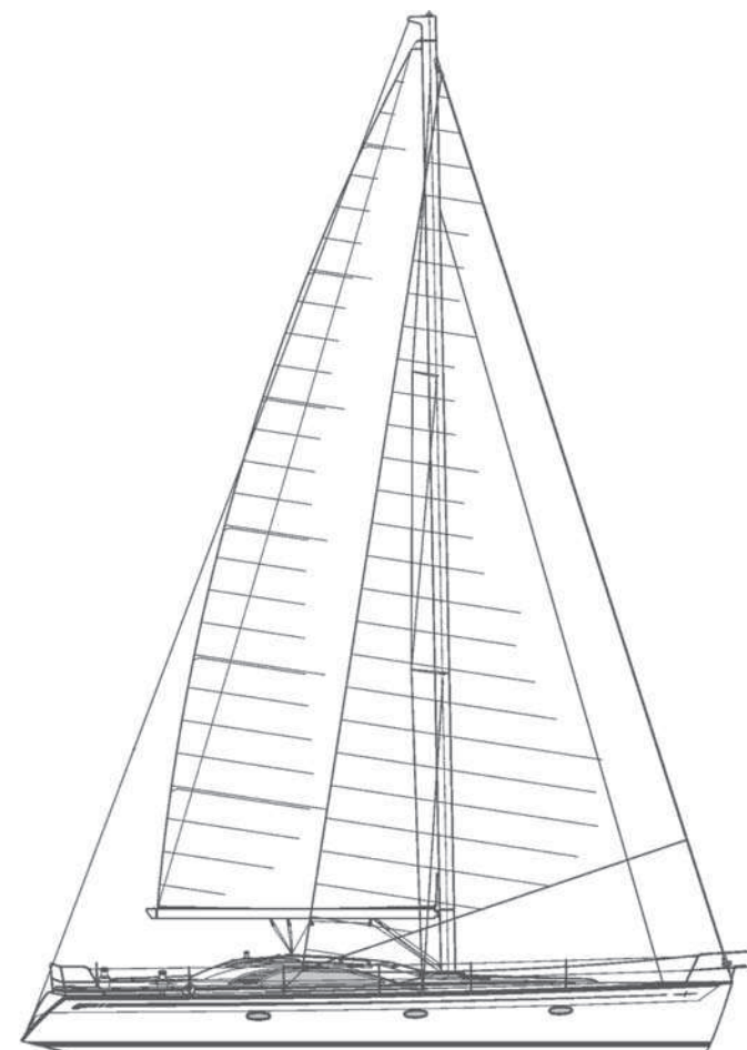
Der Segelplan./The sail plan.
